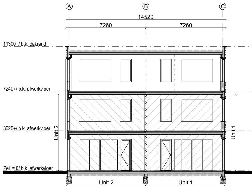
Doorsnede C-C 1:200
