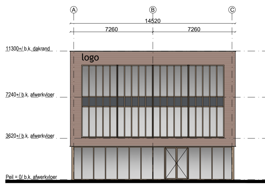
Rechterzijgevel 1:200
